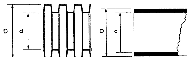
FIG. 54 - Tubi termoplastici di tipo leggero (L) e pesante (P) - Diametri
