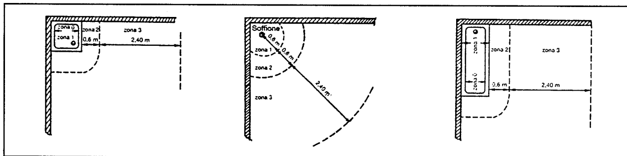
FIG. 6 - Locali bagni e docce - Zone di rischio
